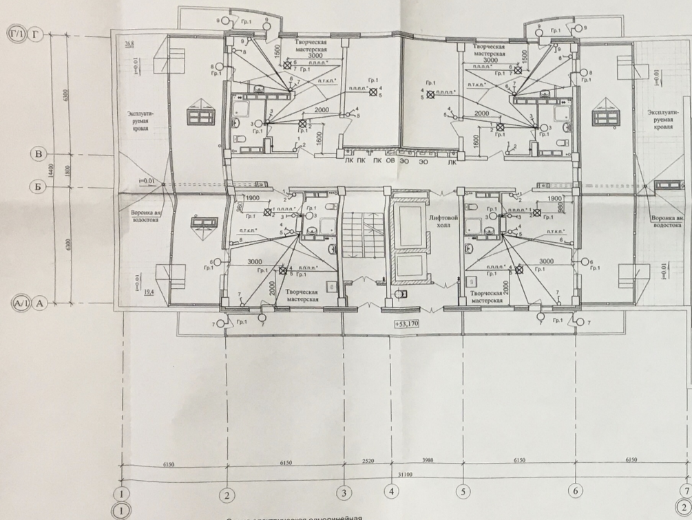
Схема электрическая однолинейная электроснабжения квартиры
