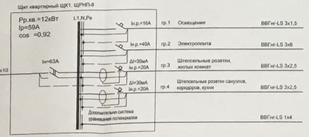
Схема электрическая однолинейная электроснабжения квартиры
