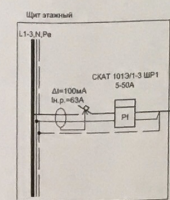
Схема электрическая однолинейная электроснабжения квартиры
