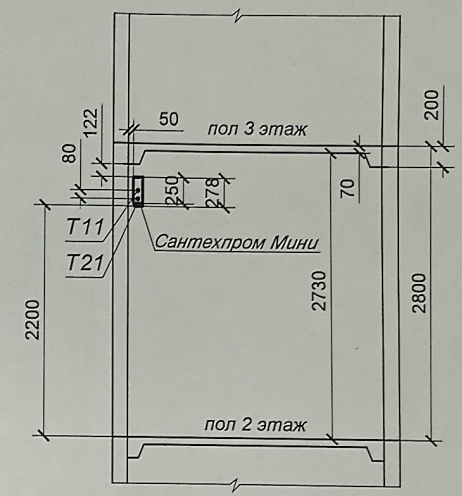
Обвязка прибора отопления на лестничной клетке
