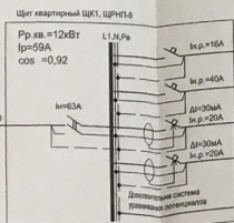
Схема электрическая однолинейная электроснабжения квартиры
