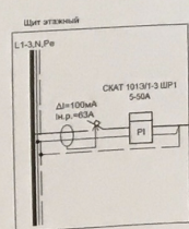
Схема электрическая однолинейная электроснабжения квартиры
